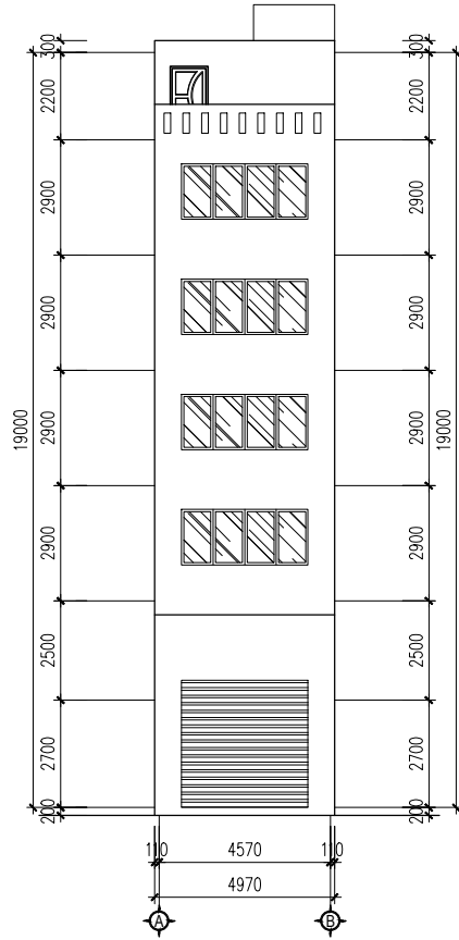
MẶT ĐÚNG CÔNG TRÌNH ĐÃ ĐƯỢC CẤP PHÉP XÂY DỰNG
