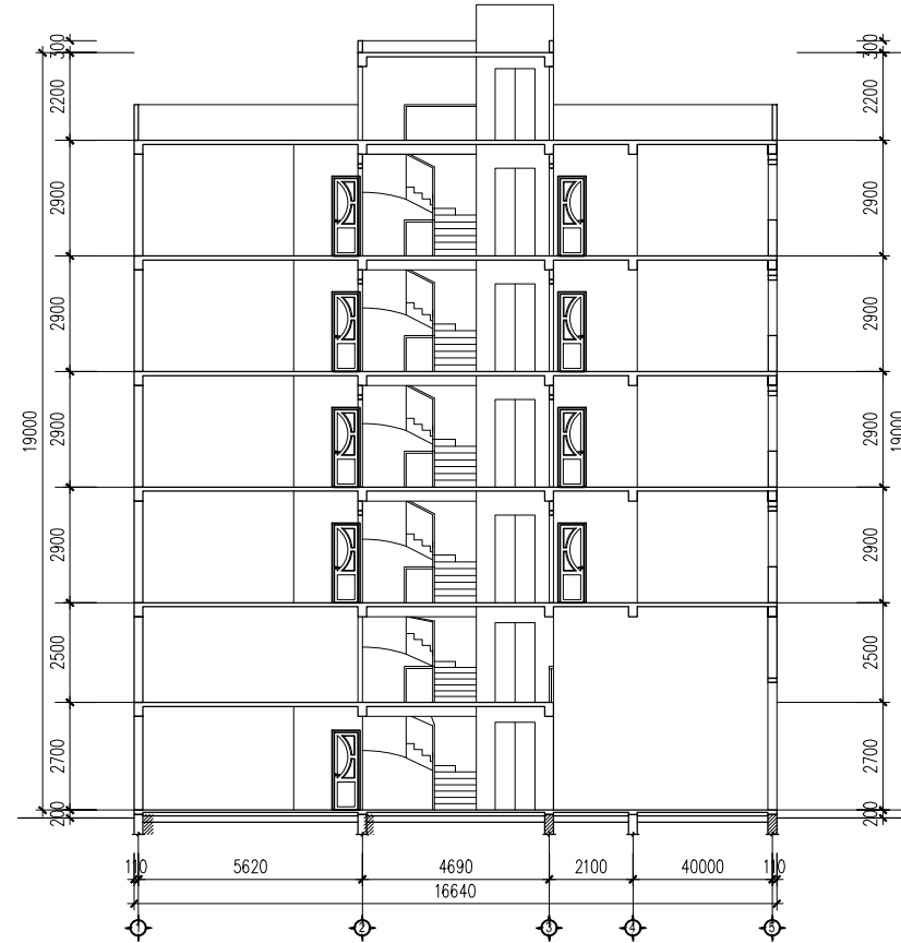
MẶT CẮT CÔNG TRÌNH ĐÃ ĐƯỢC CẤP PHÉP XÂY DỰNG
